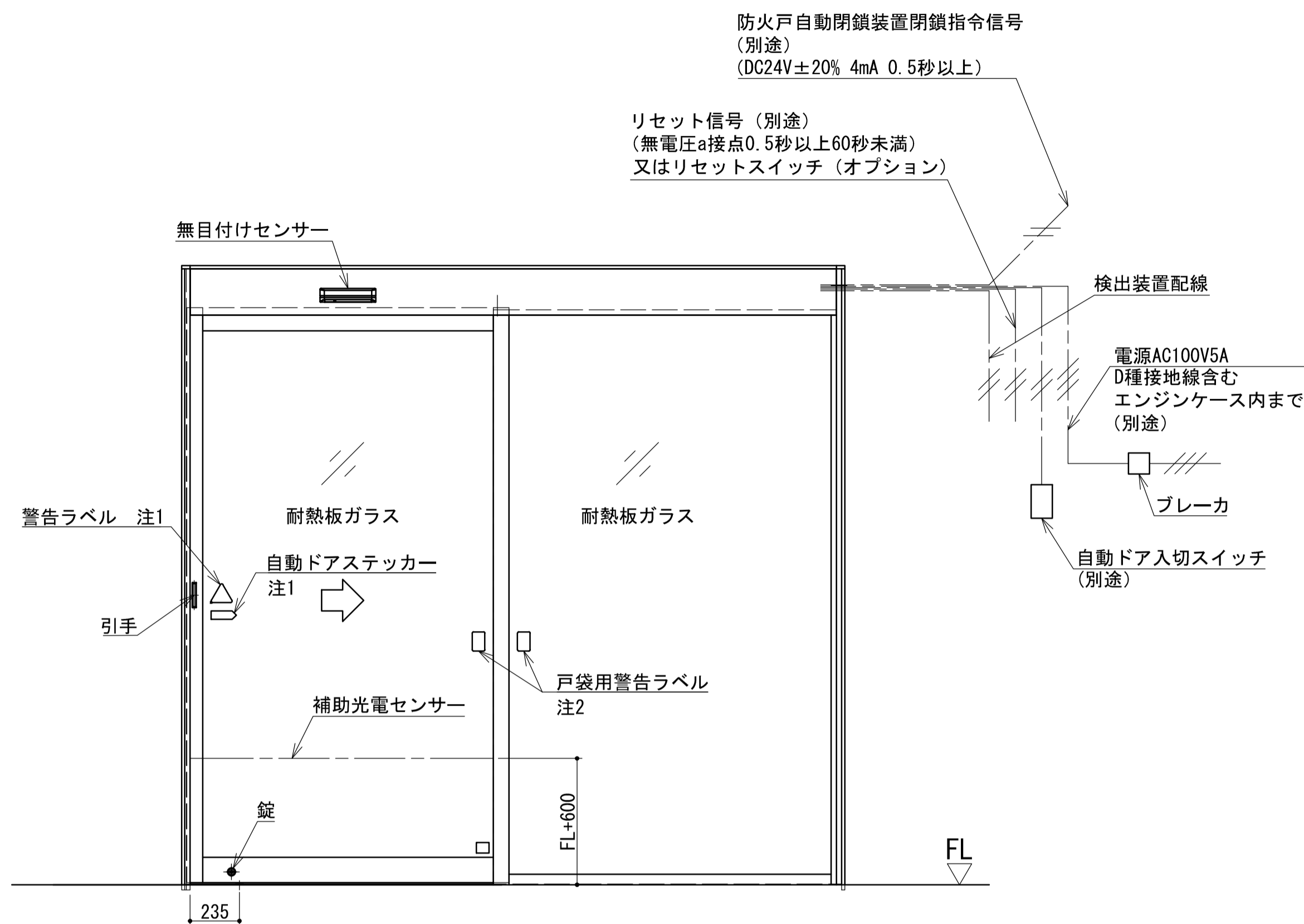
外観図 (右勝手)
