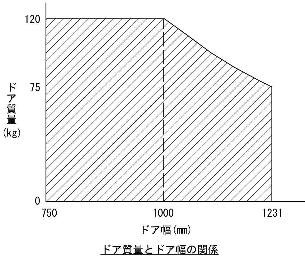
ドア質量とドア幅の関係
