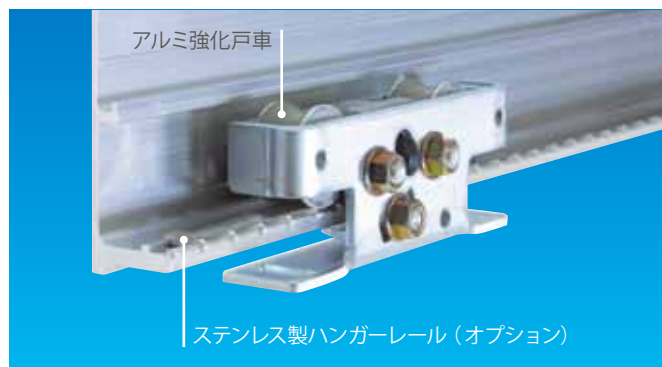
強度アップしたドア支持機構 (DSN-250 は構造が異なります。)
