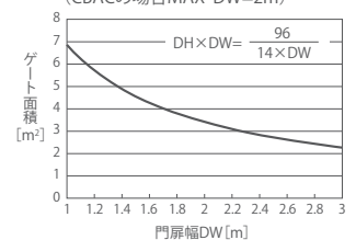
422SBS・CBAC適用ゲート受圧面積 (CBACの場合MAX DW=2m)
