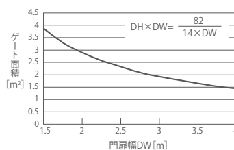
415適用ゲート受圧面積
